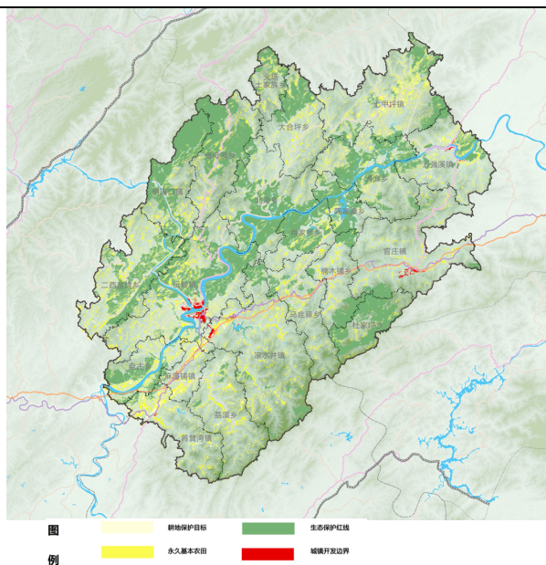
图 3-1 沅陵县控制线规划图
