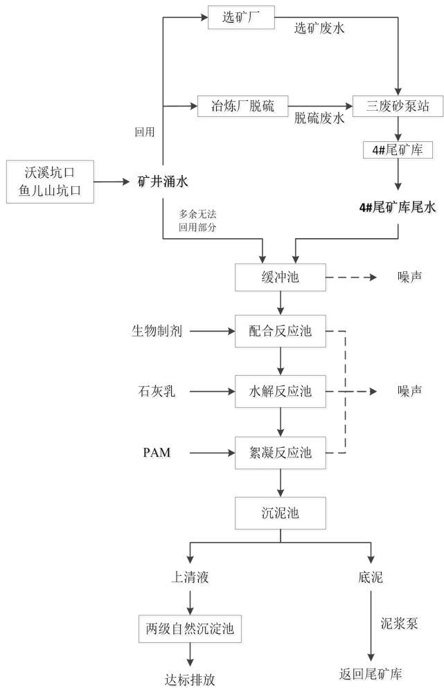
图2-1 本项目运营期工艺流程图
