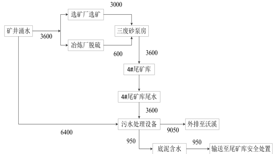
图 2-2 项目水平衡图 单位：m³/d
