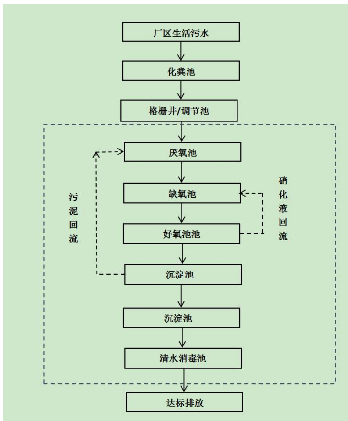
图2-2 本项目生活污水工艺流程图
