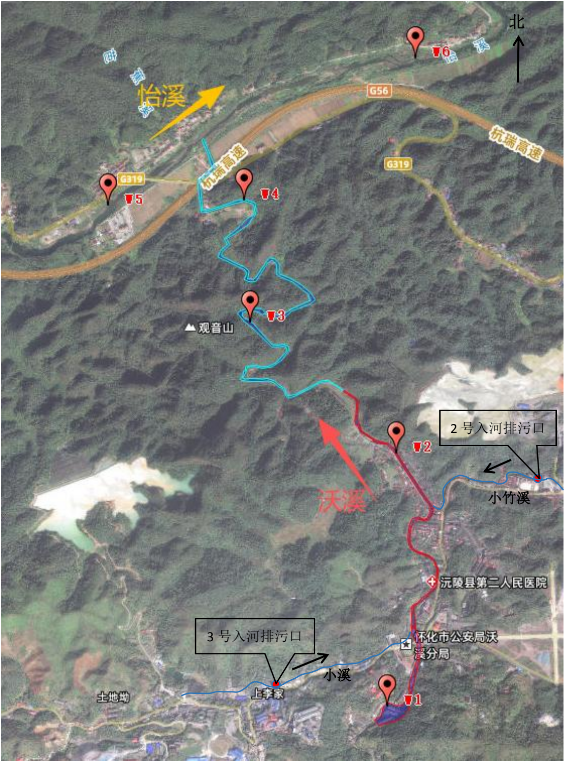
图3.1-2 沃溪地表水水质监测断面布设情况表
