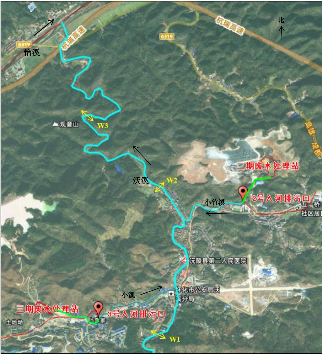
图 3.2-1 沃溪地表水水质监测断面布设情况图
